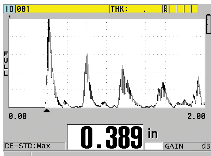
室外显示设置, A扫描模式
