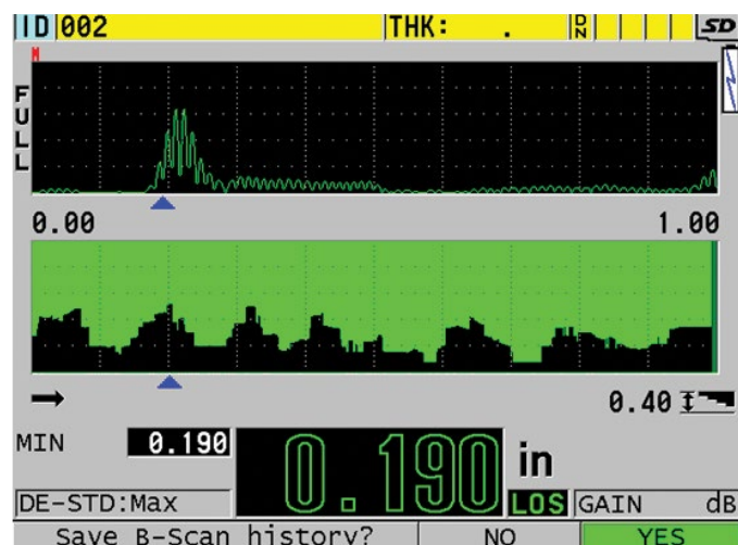
室内显示设置, B扫描模式
